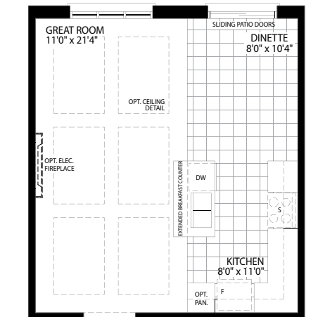
OPTIONAL MAIN FLOOR ELEV. A
